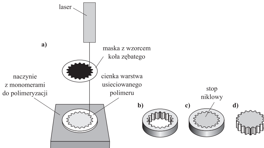
Rys. 27.7. Otrzymywanie mikrokoła zębatego za pomocą stereolitografii, a) naświetlanie mieszaniny polimeryzującej za pomocą lasera poprzez maskę ze wzorcem koła zębatego, b) końcowa forma gotowego spolimeryzowanego obiektu, c) wypełnienie formy stopem niklu metodą elektroformowania, d) końcowy produkt – mikrokoło zębate.
