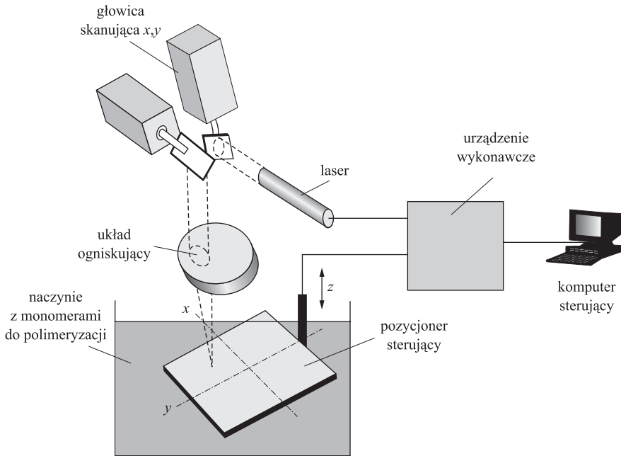
Rys. 27.6. Aparatura do stereolitografii
